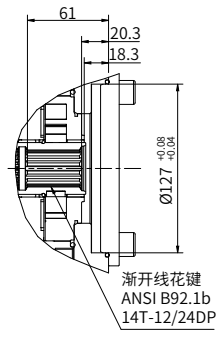
“C2” 型通轴驱动
