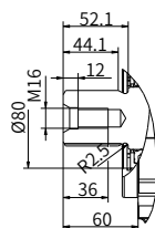
“CE” 型花键轴
