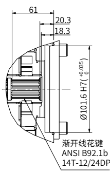
“B4” 型通轴驱动
