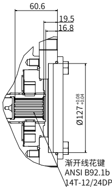
“C6” 型通轴驱动
