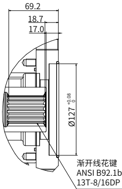
“CF” 型通轴驱动
