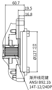
“CC” 型通轴驱动
