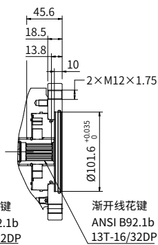
“B1”型通轴驱动
