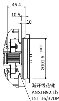
“B3”型通轴驱动
