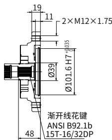
“B3” 型通轴驱动
