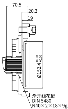
“D4”型通轴驱动
