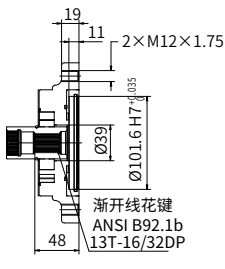
“B1” 型通轴驱动
