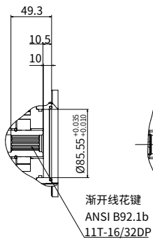
“A2”型通轴驱动
