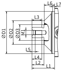
“A” 型输入轴
