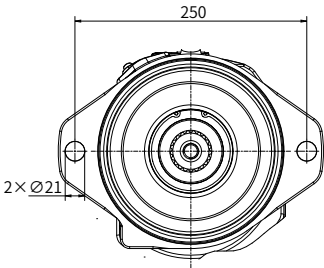
“S2” 型法兰 ISO 3019-2 200-2
