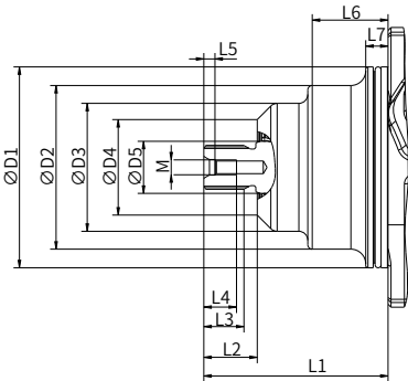
“B” 型输入轴
