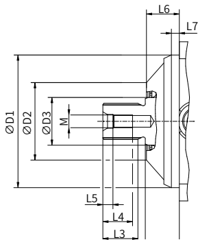
“B” 型输入轴
