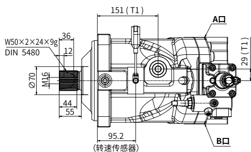
Y向视图
