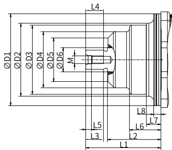
“B” 型输入轴
