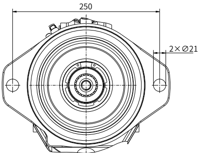
“S2” 型法兰 ISO 3019-2 200-2
