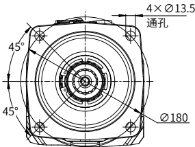
“N4” 型法兰 ISO 3019-2 140-4
