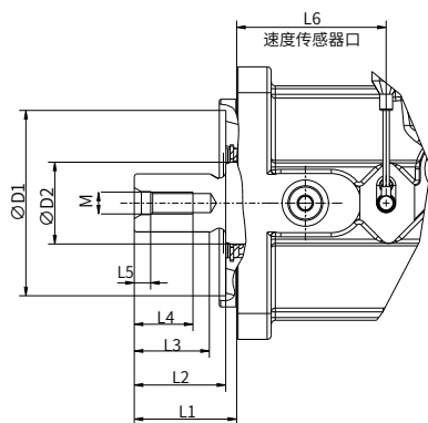
“A3”型输入轴
