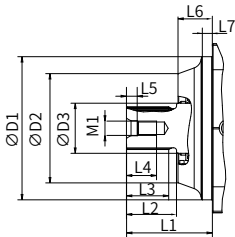
“A” 型输入轴
