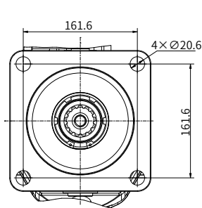
“D4” 型法兰 SAE J744 152-4
