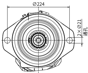
“Y2” 型法兰 ISO 3019-2 190-2
