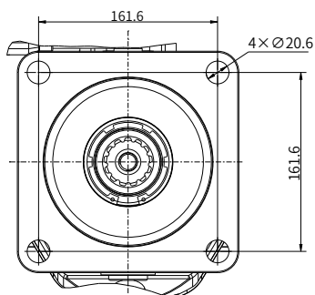
“D4” 型法兰 SAE J744 152-4
