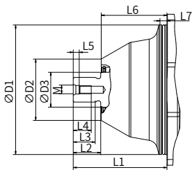
“A2” 型输入轴
