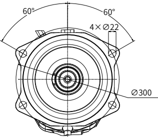
“E4” 型法兰 ISO 3019-2 260-4
