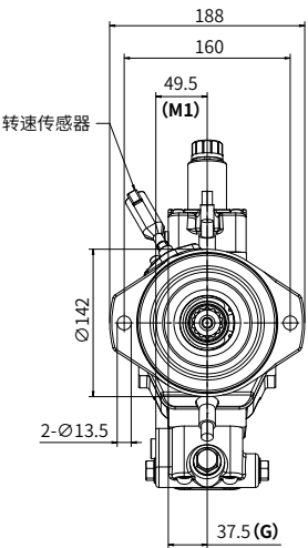
X向视图
