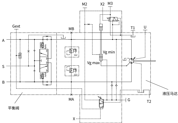
平衡阀 (带第二小排量)
