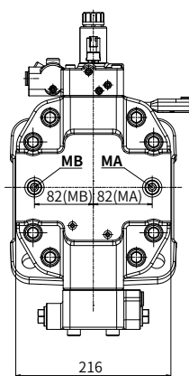
Z向视图
