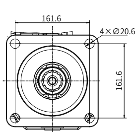
“D4” 型法兰 SAE J744 152-4
