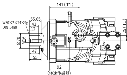
Y向视图
