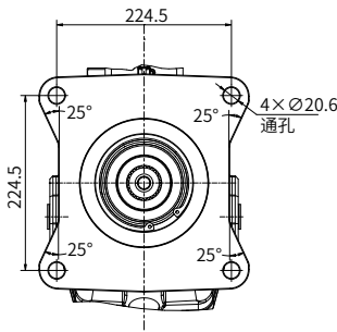
“T4” 型法兰 SAE J744 165-4
