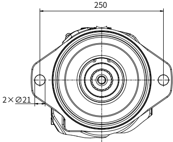
“S2” 型法兰 ISO 3019-2 200-2
