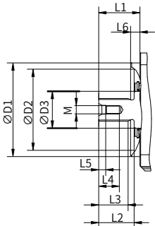
“S” 型输入轴
