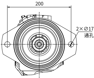
“P2” 型法兰 ISO 3019-2 160-2
