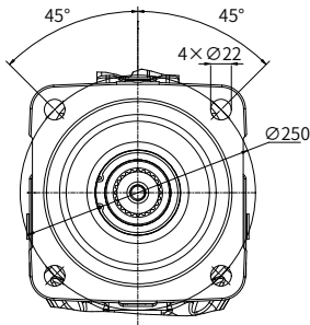
“S4” 型法兰 ISO 3019-2 200-4
