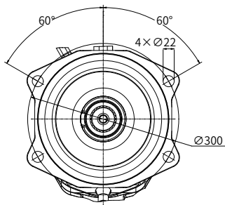
“E4” 型法兰 ISO 3019-2 260-4
