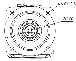
“M4” 型法兰 ISO 3019-2 125-4
