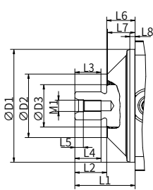
“A” 型输入轴
