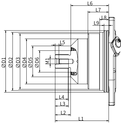
“A” 型输入轴
