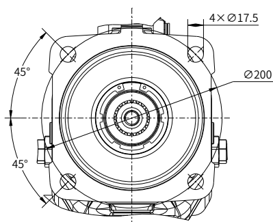
“P4” 型法兰 ISO 3019-2 160-4
