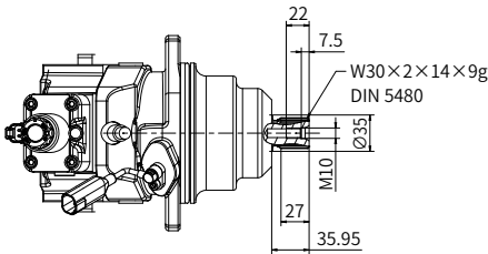
Y向视图
