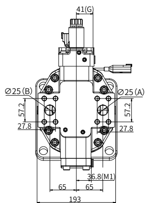
Z向视图
