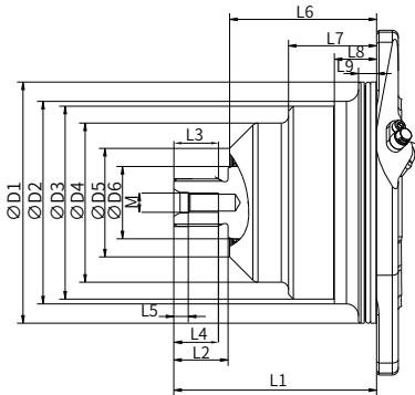
“B” 型输入轴
