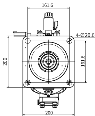
X向视图
