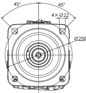
“S4” 型法兰 ISO 3019-2 200-4
