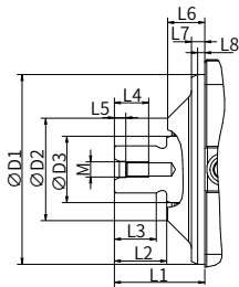
“S4” 型法兰 ISO 3019-2 200-4
