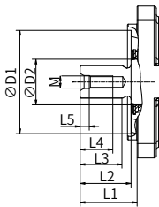
“A3” 型输入轴
