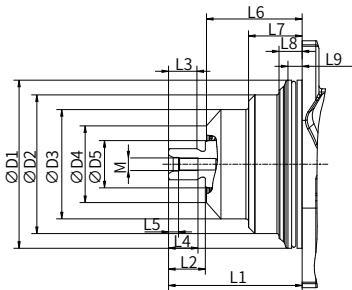
“B” 型输入轴
