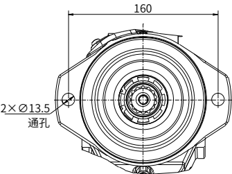
“L2” 型法兰 ISO 3019-2 135-2
