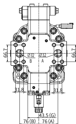
Z向视图
