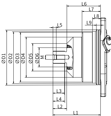
“A” 型输入轴
