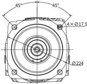
“R4” 型法兰 ISO 3019-2 180-4
