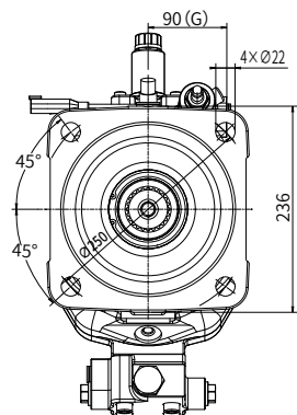
X向视图
