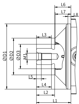
“B9” “A1” “B1” “B4” 型输入轴
