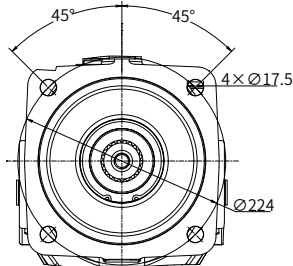
“R4” 型法兰 ISO 3019-2 180-4
